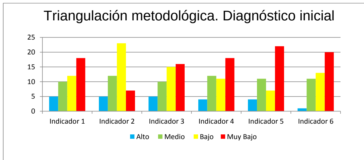
Gráfico 1.3 Triangulación metodológica
